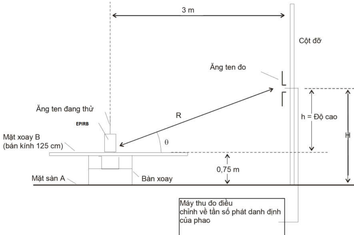
Hình 2 - Thiết lập đo kiểm
