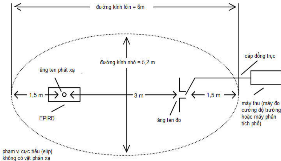
Hình 1 - Vị trí đo kiểm mẫu
