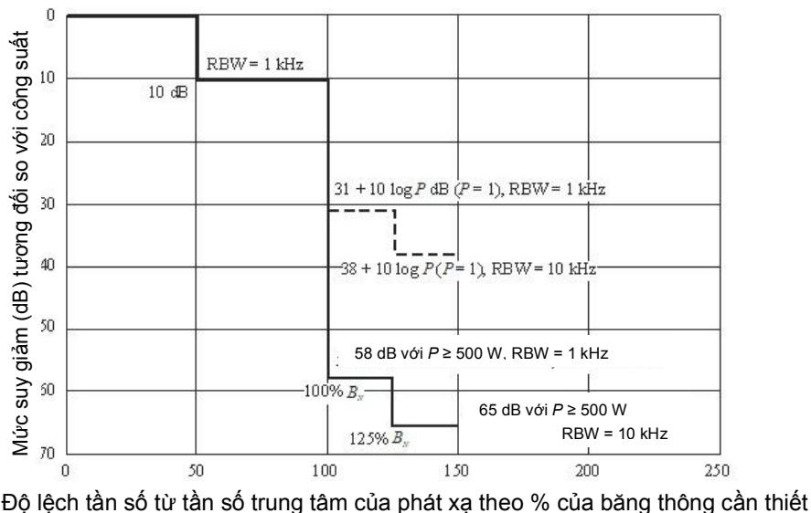
Hình D.11 - Các dải hoạt động trong dải tần trên 30 MHz trong trường hợp băng rộng của khuyến nghị ITU-R SM.1539
