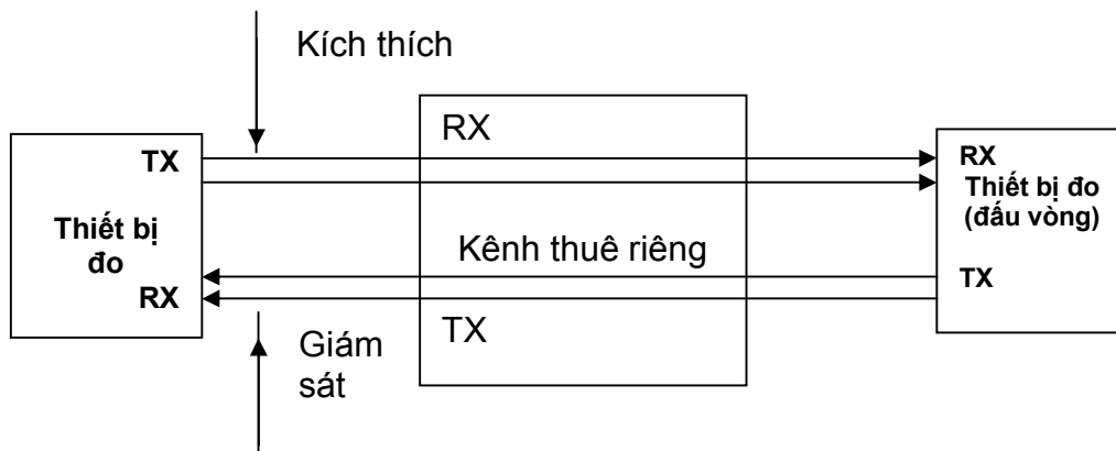
Hình 7 - Cấu hình đo trễ
