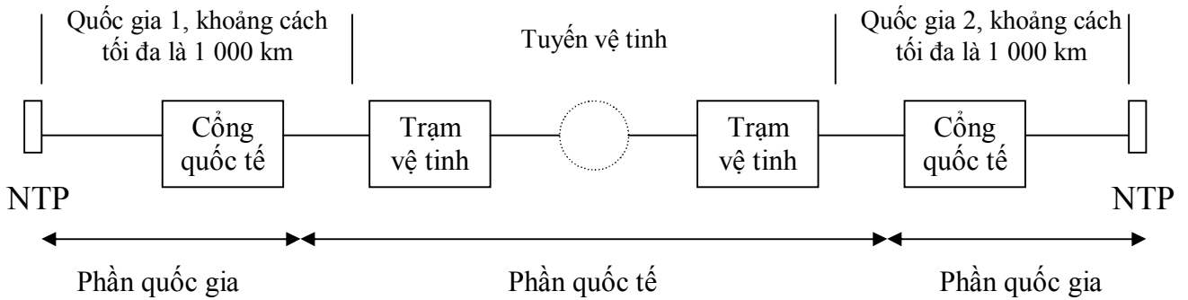
Hình A.2 - Đường truyền chuẩn cho kênh thuê riêng VC qua vệ tinh
