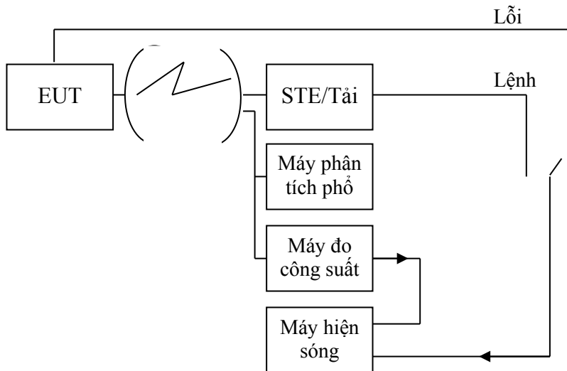
Hình 11 - Sơ đồ đo chung cho các phép đo về giám sát và điều khiển đối với những phép đo truyền dẫn
