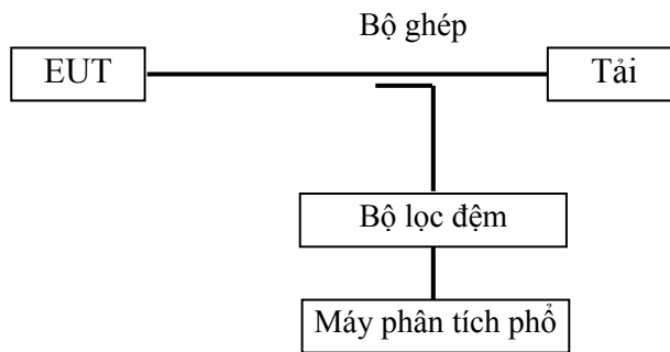
Hình 6 - Sơ đồ đo bức xạ tạp trên trực tại mặt bích anten
