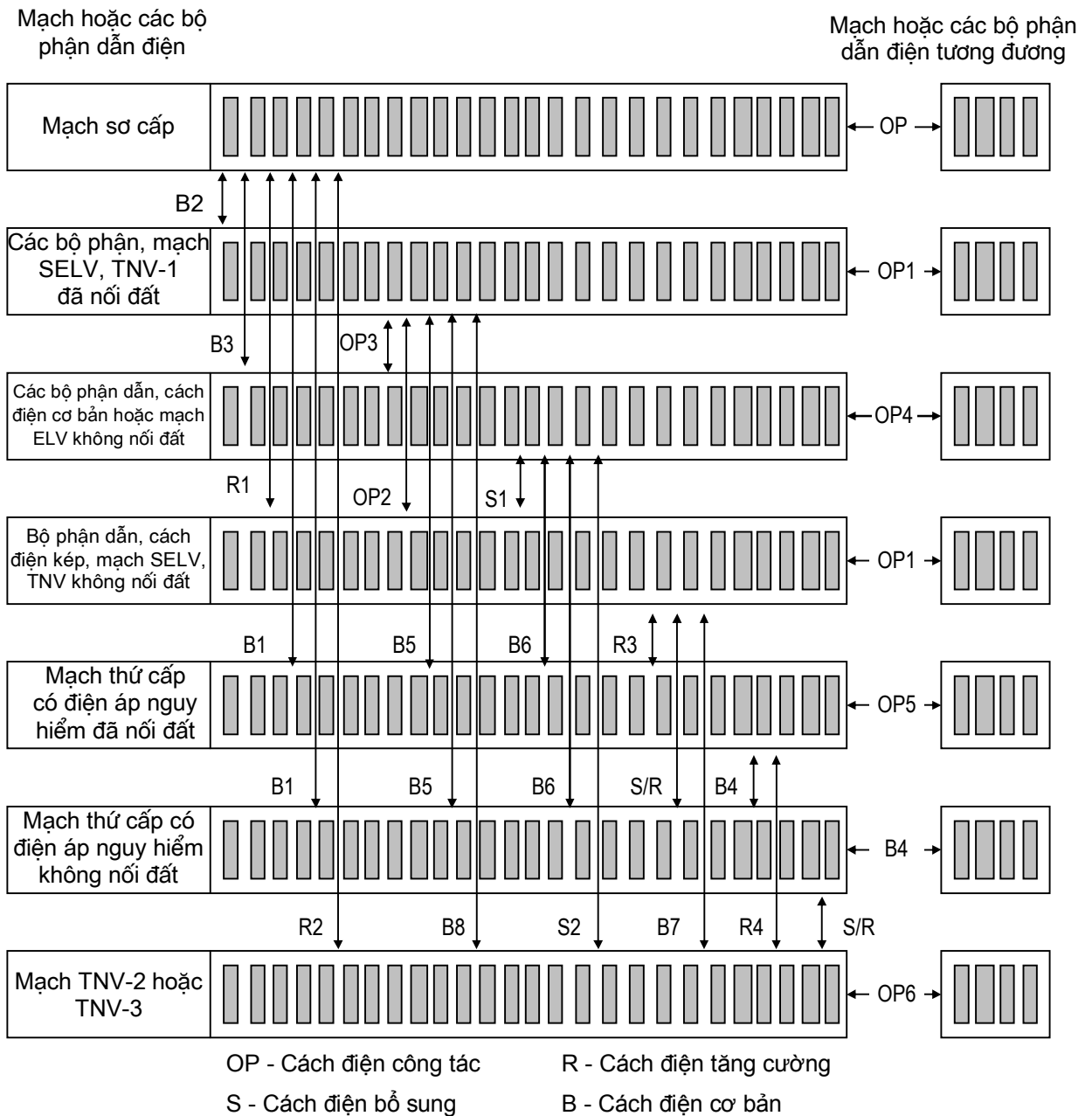
Hình 7 - Các ví dụ về việc ứng dụng của lớp cách điện
