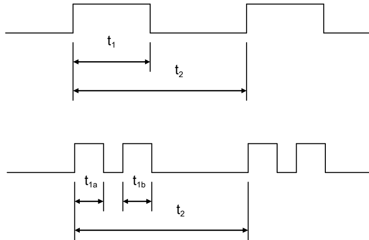
Hình C.1 - Độ rộng và chu kỳ tín hiệu chuông
