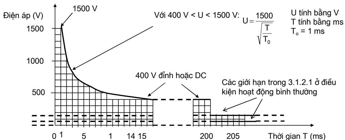
Hình 1 - Điện áp cực đại mạch TNV sau khi có một hồng đơn
