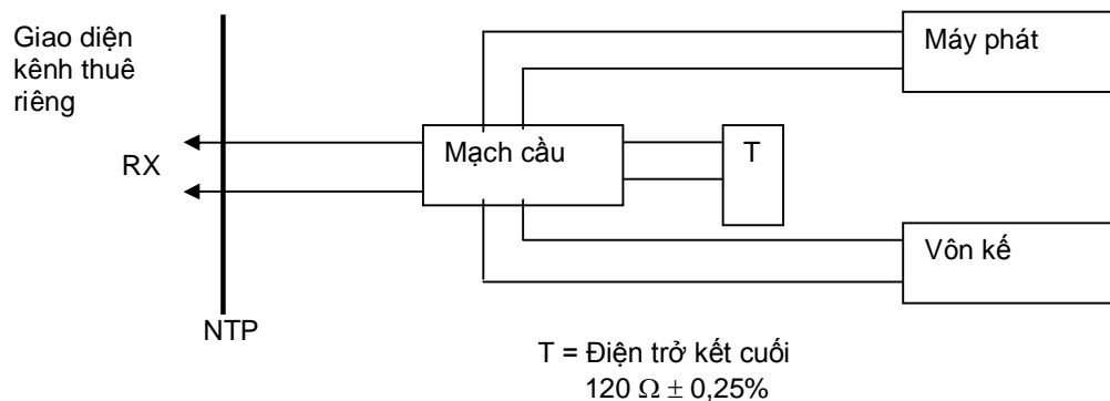
Hình A.3 - Suy hao phản xạ ở lối vào
