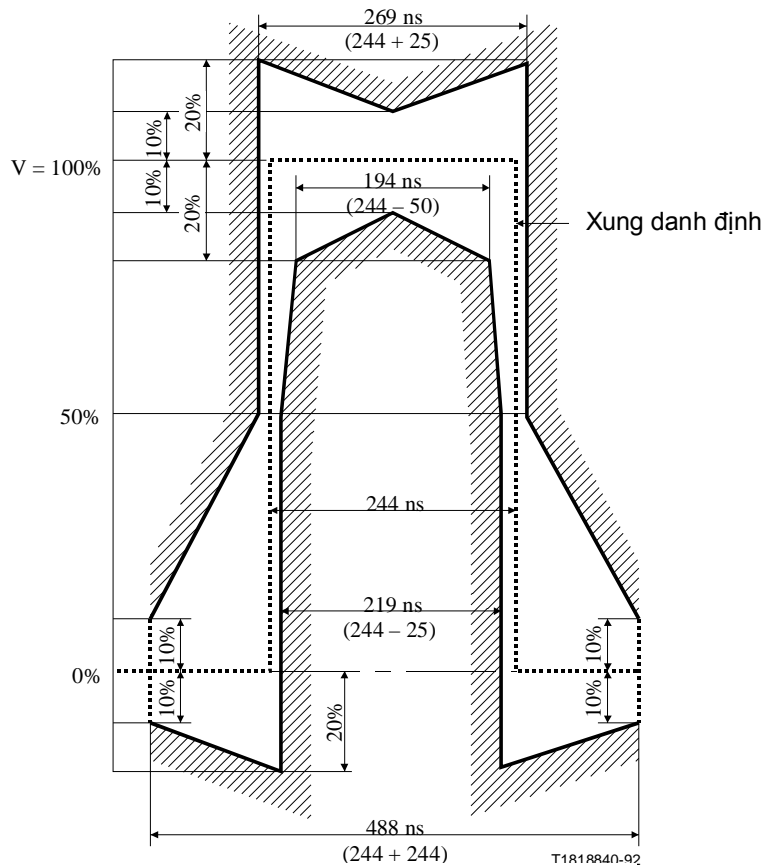
CHÚ THÍCH: V là giá trị đỉnh danh định
