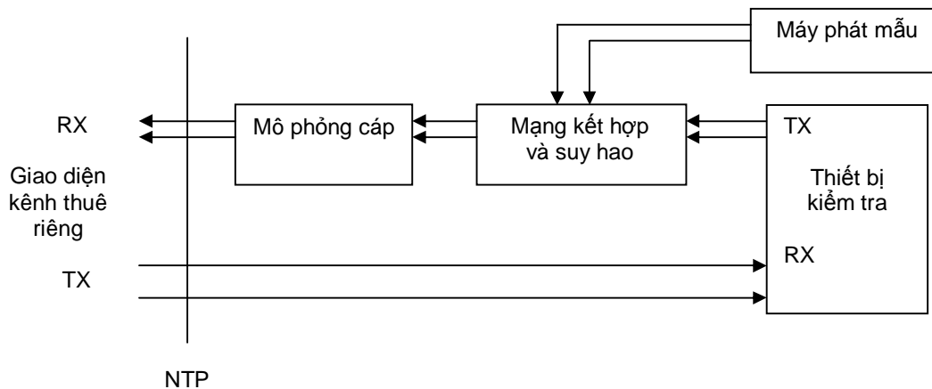
Hình A.4 - Miễn nhiễm với phản xạ
