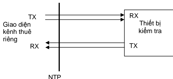
Hình A.1 - Mã hoá tín hiệu cổng lối ra
