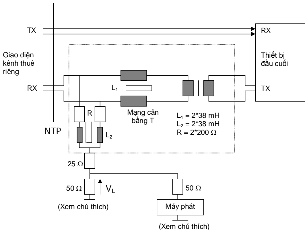
Hình A.5 - Khả năng chịu điện áp dọc, việc mã hoá lối vào HDB3
