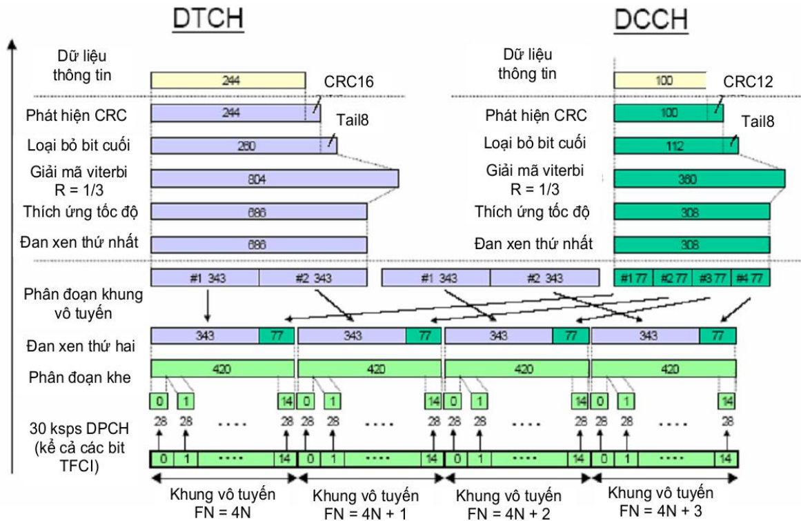
Hình D.1.1 - Mã hoá kênh đo tham chiếu DL (12,2 kit/s)
