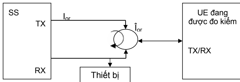
Hình C.1 - Sơ đồ đo kiểm TX cơ bản
