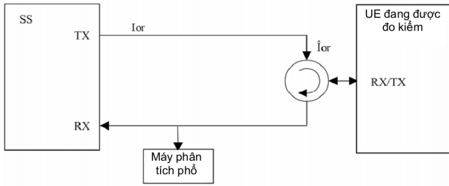
Hình C.6 - Sơ đồ đo kiểm phát xạ giả
