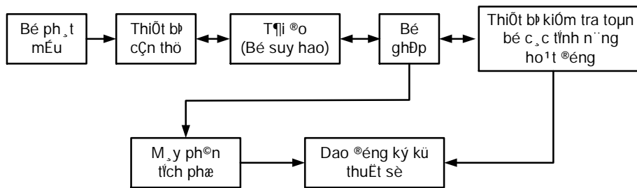
Hình 19 - Sơ đồ đo định thời phát b)
