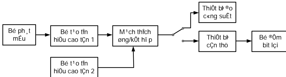
Hình 24 - Sơ đồ đo các miễn nhiễm đáp ứng tạp
