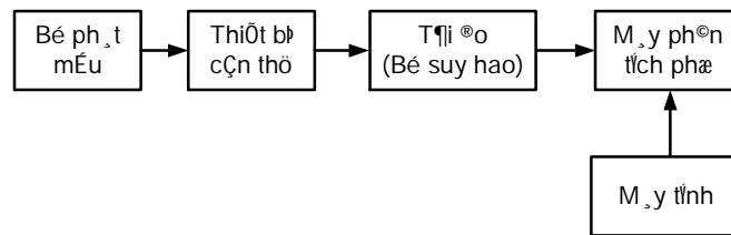
Hình 9 - Sơ đồ đo băng tần chiếm dụng
