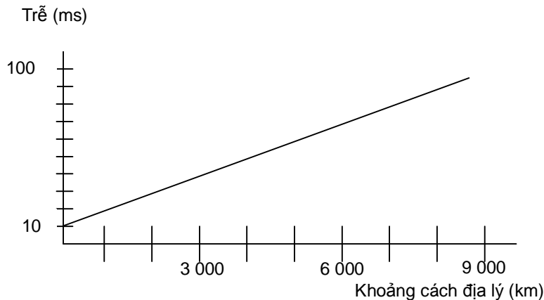
Hình 1 - Giới hạn trên của trễ truyền dẫn
