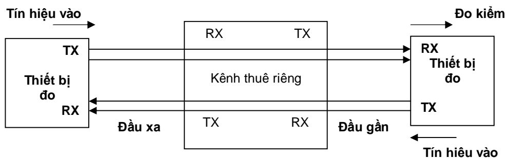
Hình A.6 - Đo cấu trúc khung
