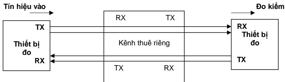
Hình A.3 - Đo rung pha
