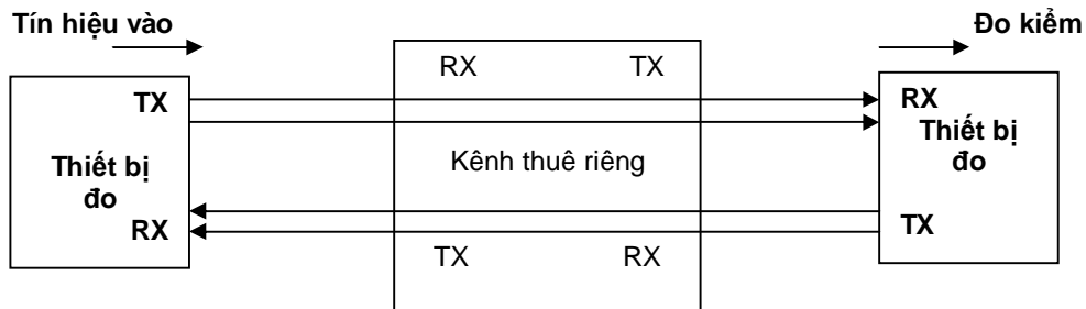
Hình A.5 - Đo lỗi và trượt
