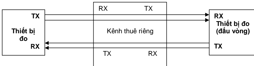
Hình A.2 - Cấu hình đo trễ
