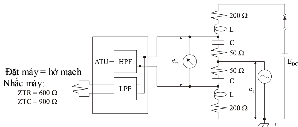
Hình 6 - Phương pháp đo cân bằng dọc trong dải tần lớn hơn 30 kHz (HPF và LPF được tích hợp trong ATU)
