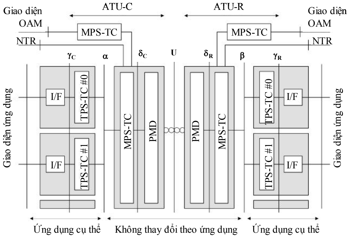
Hình 1 - Mô hình chức năng của ATU
