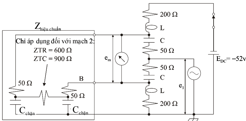
Hình 7 - Mạch hiệu chuẩn
