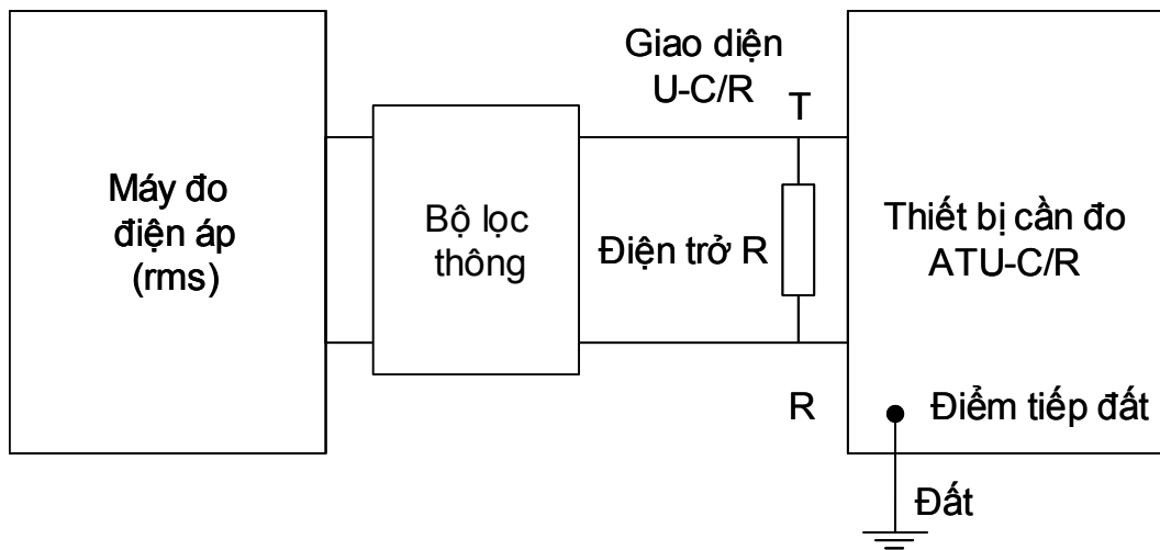
Hình 10 - Cấu hình đo tổng công suất phát
